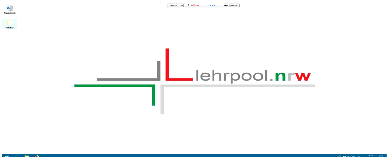
Abbildung 0.4: PVS* Teilnahme
