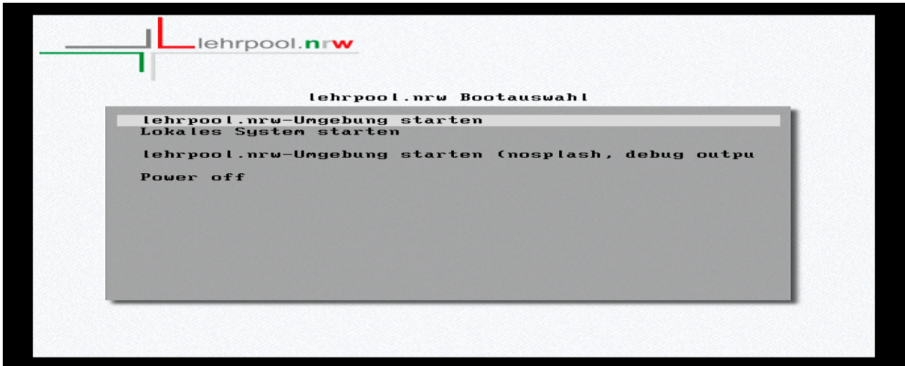
Abbildung 0.1: lehrpool.nrw Bootauswahl
