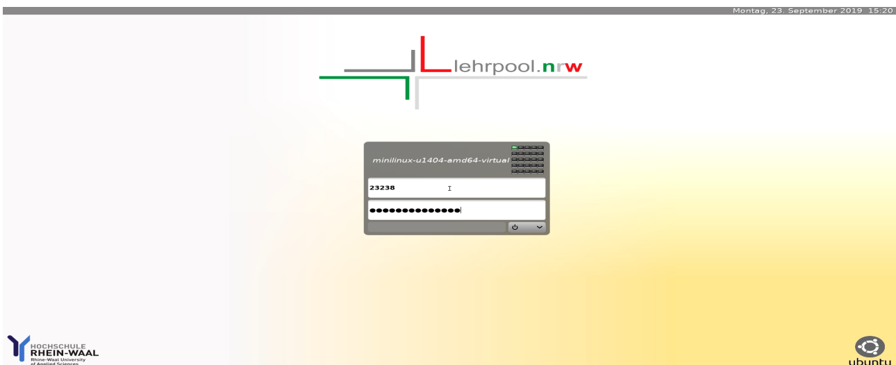
Abbildung 0.2: lehrpool.nrw Loginmaske
